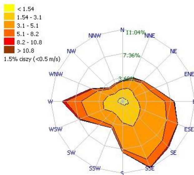
Rysunek 10. Dominujący kierunek wiatru (róża wiatrów) wyznaczony dla stacji pomiarowej Warszawa - Targówek w 2014 r. (źródło: Roczna ocena jakości powietrza w województwie mazowieckim - raport za 2014 r. WIOŚ Warszawa, 2015)
