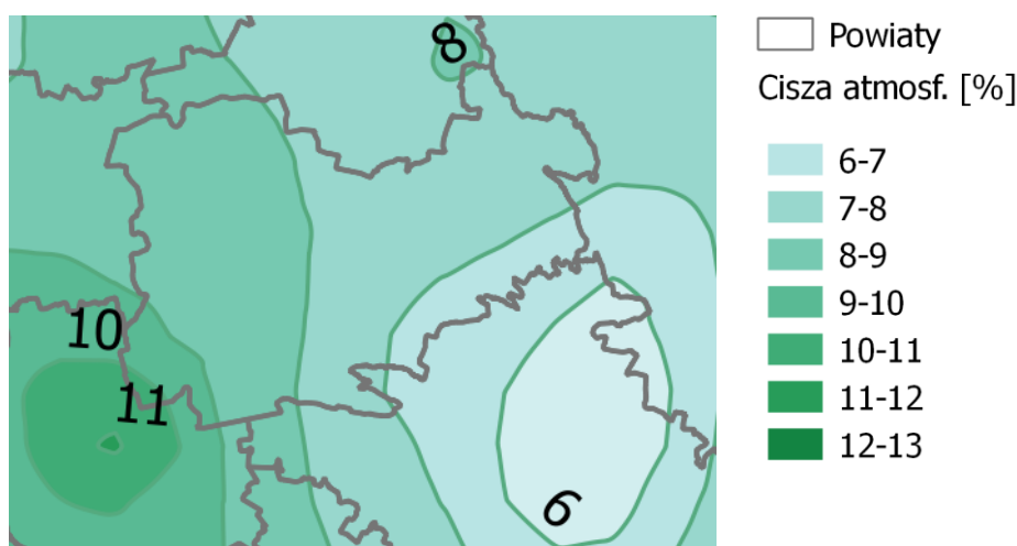
Rysunek 11. Cisza atmosferyczna w 2014 r. (źródło: Roczna ocena jakości powietrza w województwie mazowieckim - raport za 2014 r. WIOŚ Warszawa, 2015)
