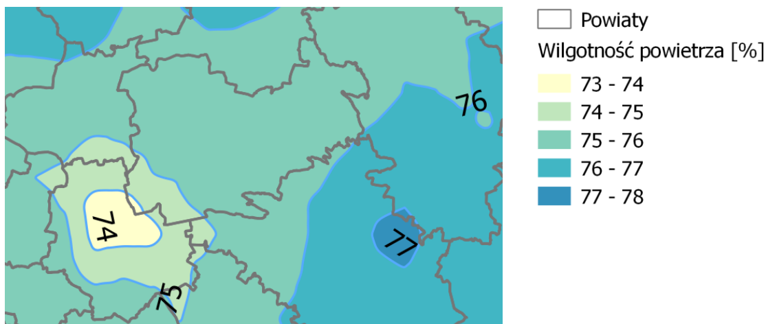
Rysunek 12. Rozkład średniej rocznej wartości wilgotności względnej powietrza w 2014 r. (źródło: Roczna ocena jakości powietrza w województwie mazowieckim - raport za 2014 r. WIOŚ Warszawa, 2015)
