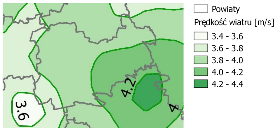
Rysunek 9. Średnia prędkość wiatru w 2014 r. (źródło: Roczna ocena jakości powietrza w województwie mazowieckim - raport za 2014 r. WIOŚ Warszawa, 2015)
