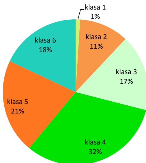
Rysunek 13. Udział klas równowagi atmosfery na wybranych stanowiskach dla stacji pomiarowej Warszawa - Targówek w 2014 r. [%] (źródło: Roczna ocena jakości powietrza w województwie mazowieckim - raport za 2014 r. WIOŚ Warszawa, 2015)
